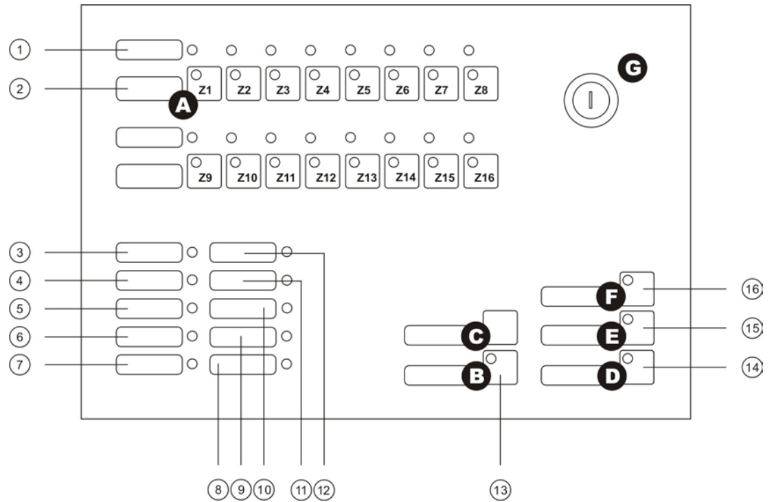
Figure 2 : Panneau avant FP404
