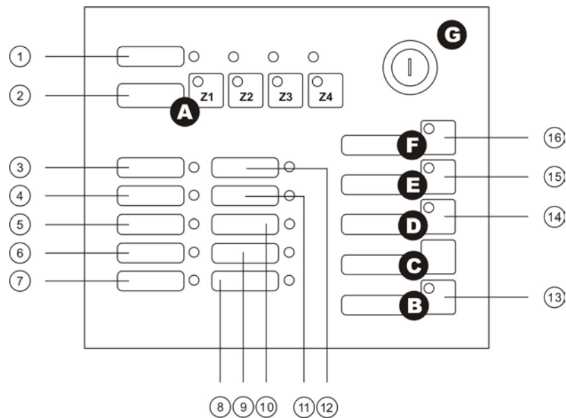
Figure 2 : Panneau avant FP404
